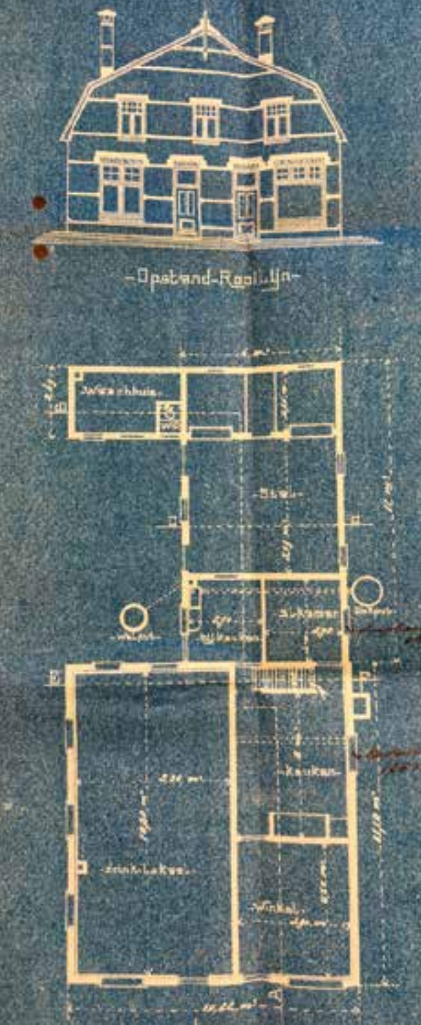
Blauwdruk bij de bouwvergunning van het café met woonhuis aan de Oudestraat.
