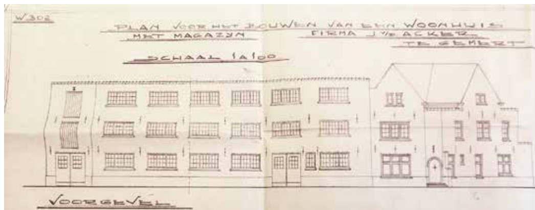
De bouwtekening uit 1935 van woning met magazijn in de Ruijschenberghstraat.
